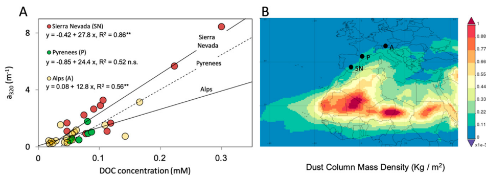
Figure 5. Concentration and absorption of dissolved organic matter in alpine lakes in Europe located in a range of distance from Saharan dust source. (A) Relationship between the DOC concentration and absorption coefficient at 320 nm ( a_{320} ) for lakes in catchments above tree line in Sierra Nevada (SN, red circles), Pyrenees (P, green circles) and Alps (A, yellow circles). Regression lines, equations and level of significance are shown. The dashed regression line indicates a no significant relationship. ** p < 0.01 ; n.s., not significant. Redrawn from Mladenov et al. (2008). (B) Location of SN, P, and A in a representative map of time-averaged dust-column mass density in \text{kg}/\text{m}^2 for a period with a Saharan dust intrusion toward the Mediterranean basin (4–21 September 2008) obtained with the second Modern-Era Retrospective analysis for Research and Applications (MERRA-2). Concentración y absorción de materia orgánica disuelta en lagos alpinos de Europa situados en un rango de distancia a la fuente de polvo sahariano. (A) Relación entre la concentración de DOC y el coeficiente de absorción a 320 nm ( a_{320} ) para lagos en cuencas por encima de la línea de árboles de Sierra Nevada (SN, círculos rojos), Pirineos (P, círculos verdes) y Alpes (A, círculos amarillos). Se muestran las líneas de regresión, las ecuaciones y el nivel de significación. La línea de regresión discontinua indica una relación no significativa. ** p < 0.01 ; n.s., no significativo. Redibujado de Mladenov et al. (2008). (B) Localización de SN, P y A en el mapa representativo de la densidad de masa de la columna de polvo promediada para un periodo con intrusión de polvo sahariano hacia la cuenca mediterránea (4-21 de septiembre de 2008) obtenido con el second Modern-Era Retrospective analysis for Research and Applications (MERRA-2).
